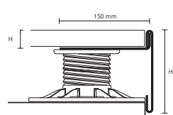
PROSUPPORT B - PROFILO TOP - ALLUMINIO VERNICIATO lunghezza barre 2,7 ml
