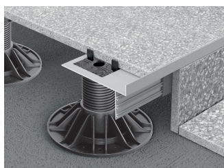
PROSUPPORT PROFILE T - ALLUMINIO TRINCIATO E VERNICIATO lunghezza barre 2,7 ml - conf. 20 Pz - 54 ml
